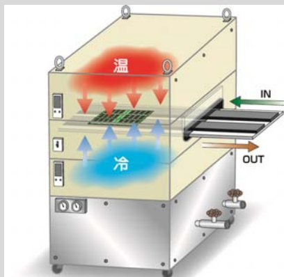
基板テストシステム用高低温試験装置
